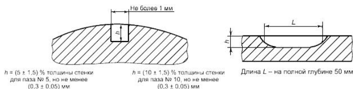
Рисунок В.1 - Виды искусственных дефектов
