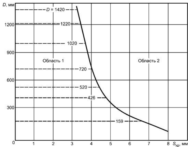
Рисунок В.3 - Графическая зависимость для настройки чувствительности дефектоскопа
