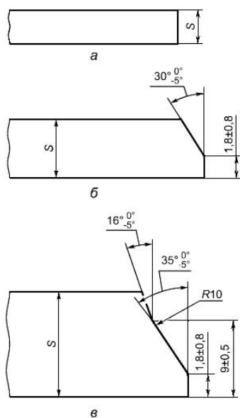
Рисунок 1 - Форма и размеры разделки торцов труб
