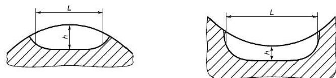
Рисунок В.2 - Виды искусственных дефектов
