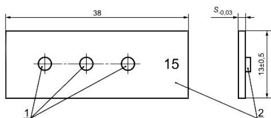
Рисунок Б.1 - Стандартный пластинчатый пенетрометр
